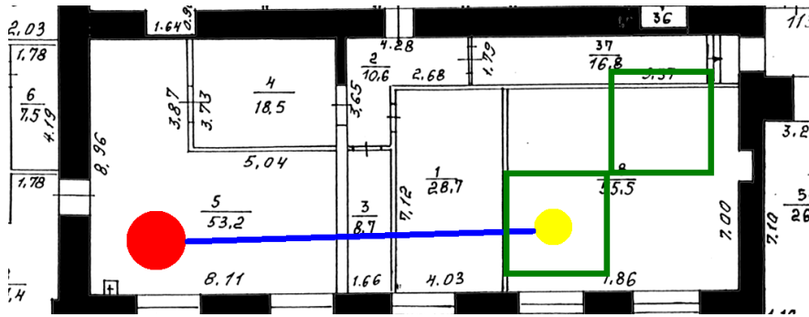
Рис. 4. Пример плана этажа для расчета. Стены – бетон.
