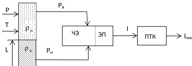
Рис. 1. Блок-схема измерительного канала уровня.
