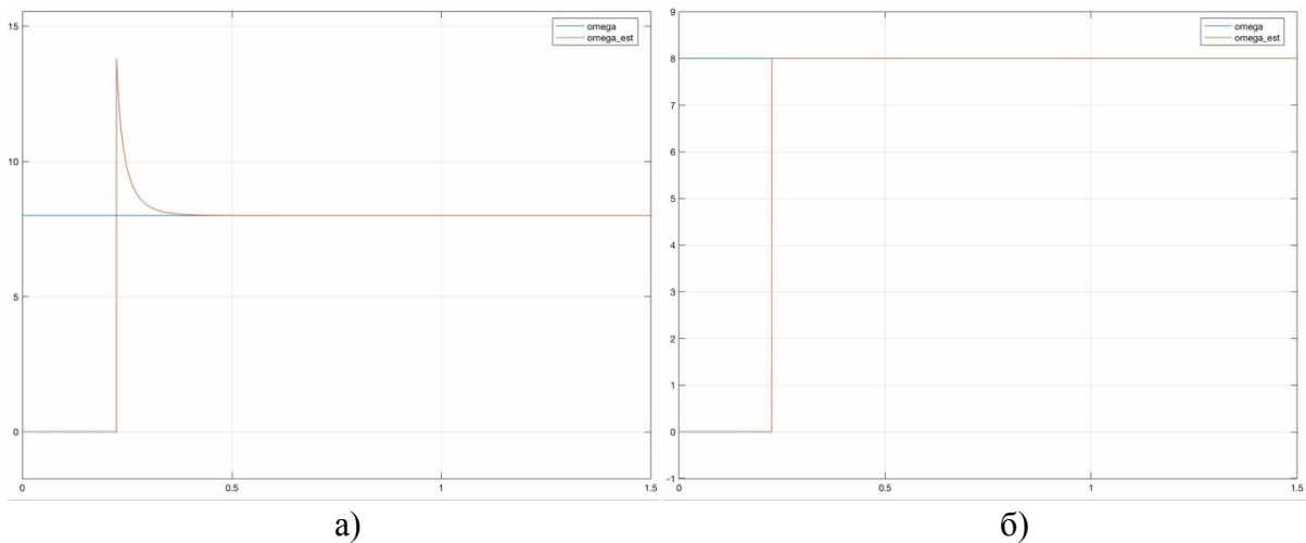
Рис. 1. Идентификация частоты сигнала (1) в отсутствии шумов измерений: а) \lambda = 30 ; б) \lambda = 120 .
