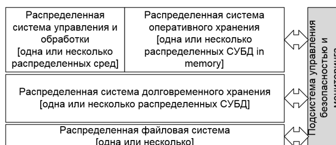
Рис. 1. Компоненты системы управления Большими данными.
