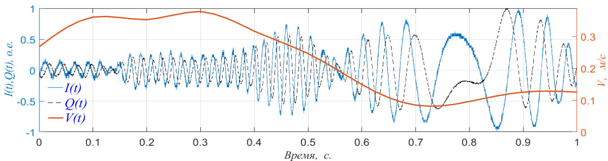
Рис. 2. Вычисление мгновенной скорости V(t) по доплеровским частотам I(t) и Q(t) СВЧ датчика.
