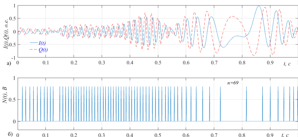
Рис. 3. Прямое вычисление перемещения а) доплеровские сигналы I_{1,2}(t) и Q_{1,2}(t) ; импульсы.
