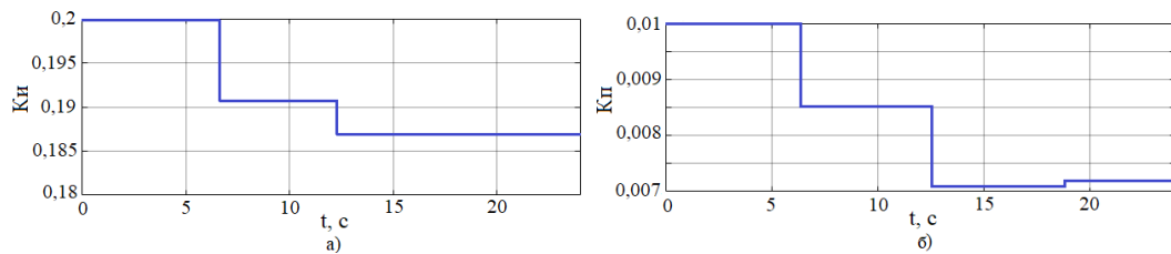
Рис. 5. Изменение K_i (а) и K_p (б) для опыта с предлагаемым нечетким настройщиком.
