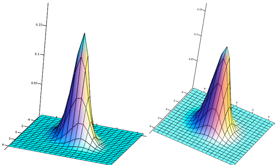
Рис. 2. Плотность распределения вероятностей f^F(z_1, z_2) из класса Фреше (слева) и двумерная гауссовская плотность распределения вероятностей с коэффициентом корреляции 1/6 (справа).
