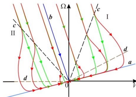
Рис. 2. Фазовые портреты системы (1) для двух форм лопастей.
