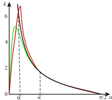
Рис. 1. Функция аэродинамического качества для прямоугольной пластины красного цвета, лопастями в форме шайбы зеленого. Функция ctg \alpha – черного цвета.
