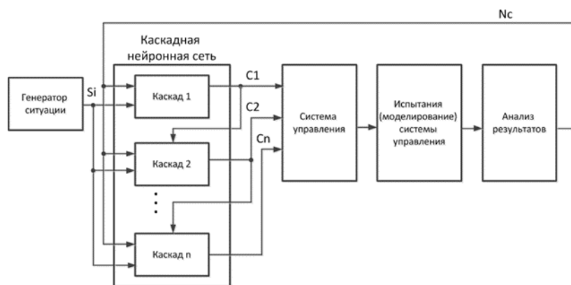
Рис. 2. Структура интеллектуальной обучающейся системы.
