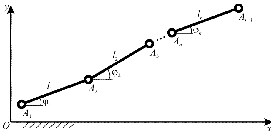
Рис. 2. Модель механизма с n подвижными звеньями переменной длины, соединенные последовательно.
