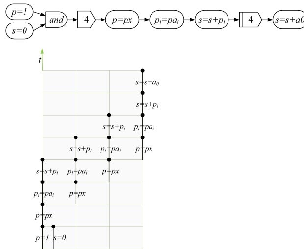
Рис. 1. Примеры графа конвейера и соответствующей временной диаграммы
