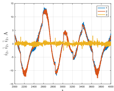
Рис. 4. Результаты идентификации модели для второго сочленения UR10
