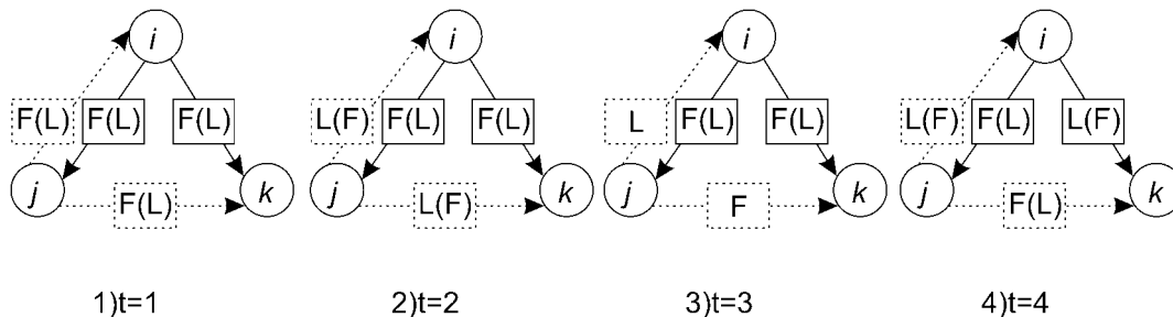
Рис. 3. Схема представлений двух рефлексирующих агентов в триполии (модель III-2).
