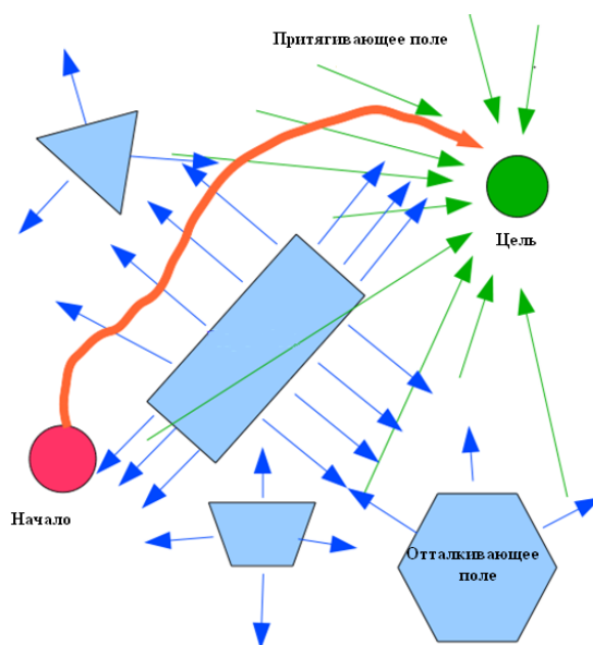
Рис. 2. Притягивающее и отталкивающие поля.
