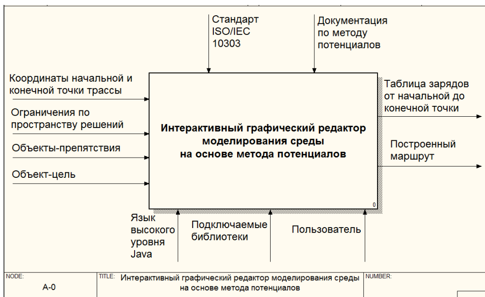
Рис. 1. Функциональная модель интерактивного редактора построения сцены.
