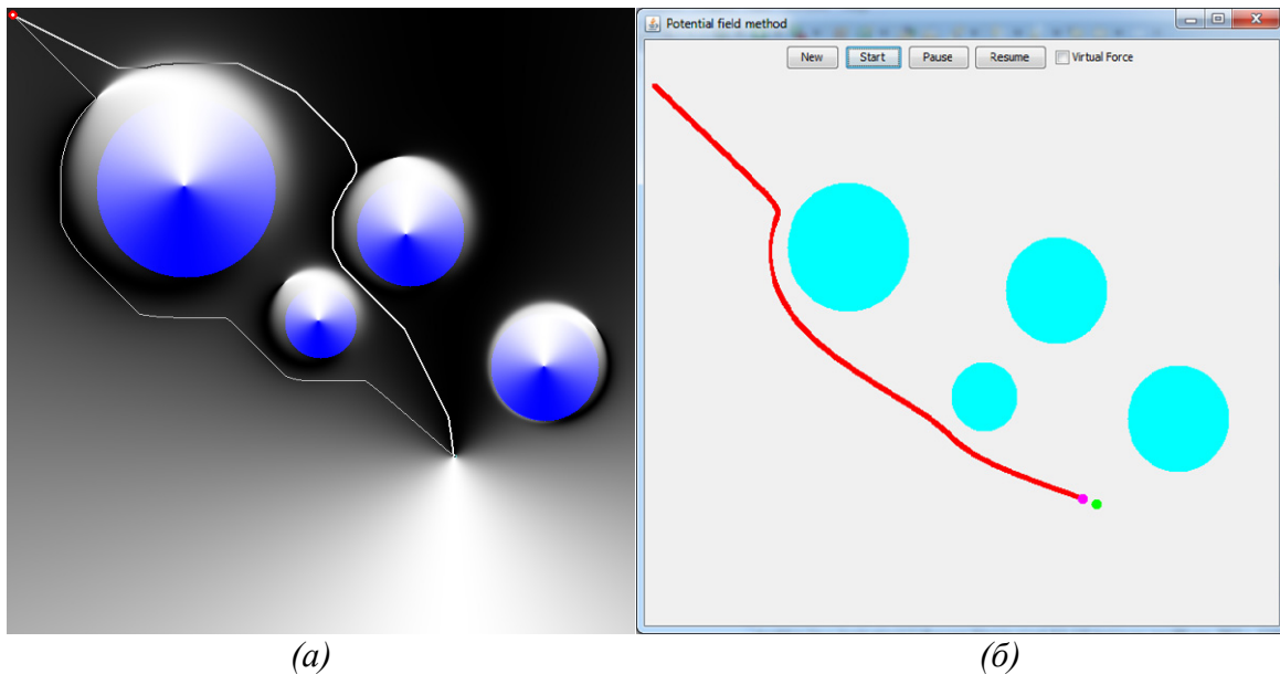
Рис. 3. Построение трассы с использованием: а) –функционально-воксельного метода; б) –метода потенциалов.
